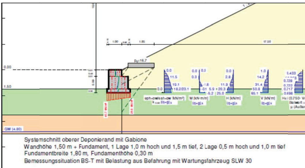
Abbildung 1: Gabionenwand, Standsicherheitsnachweis
